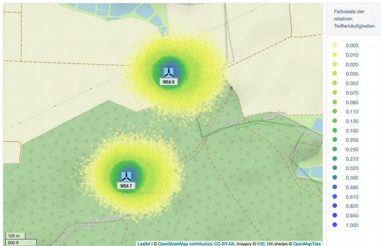
Abbildung A.1.1: Trefferhäufigkeiten von Eisstücken pro Rasterfläche (16m 2 ) und Jahr in der Umgebung der WEA 6 und 7 am Standort Neuhoﬀ Hirschneuses (Karte /1.4/).
