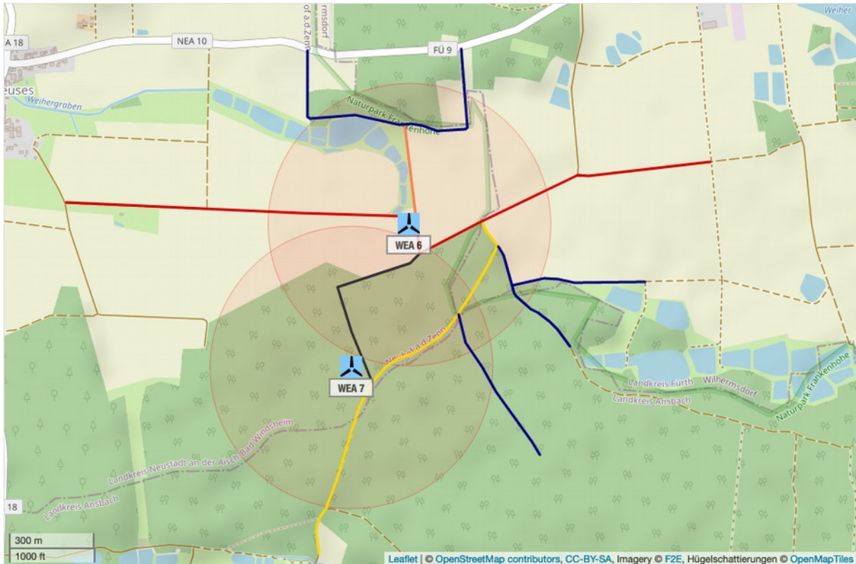
Abbildung 4.3.1: Potentielle Gefährdungsbereiche der WEA 6 und 7 und Schutzobjekte am Standort Neuhoﬀ Hirschneuses (Karte /1.4/).
